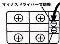
※動かさない (黒いプラスチックのネジ)
