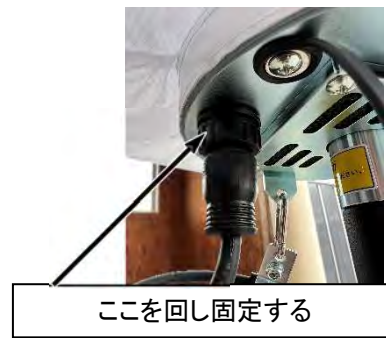
バッテリー接続用コネクタ (丸台座)
